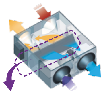
Wymiennik entalpiczny Ułatwione przenikanie wilgoci
